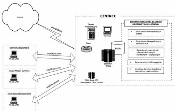
Rys. 5. Schemat Centrum Elektronicznej Informacji Regionalnej i Turystycznej
