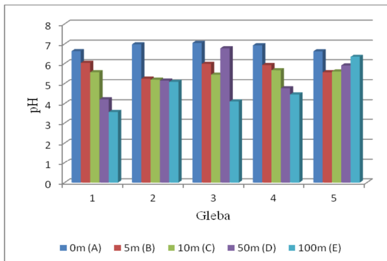
Rys. 3. Wartość pH w H 2 O w próbkach glebowych Fig. 3. The pH in H 2 O values of soil samples
