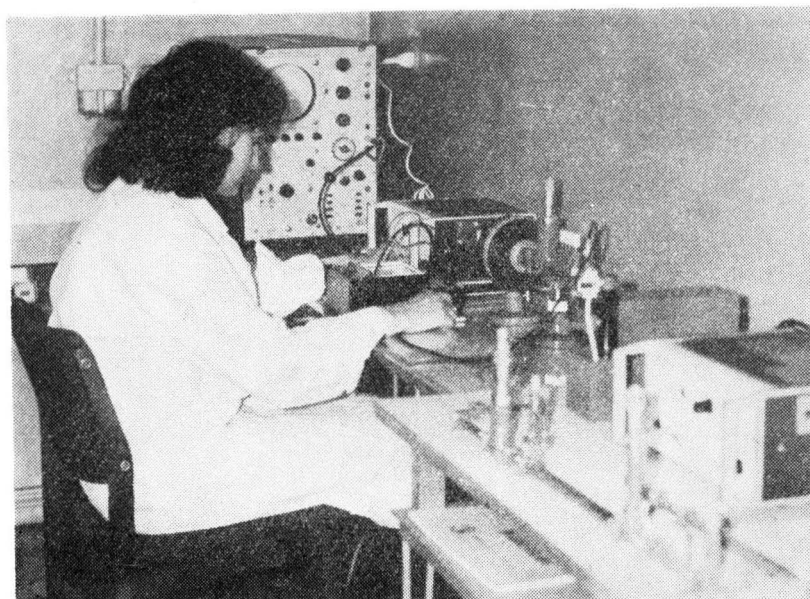
Stanowisko badań mikrofalowych w Zakładzie Fizyki foto K. Jarocińska
