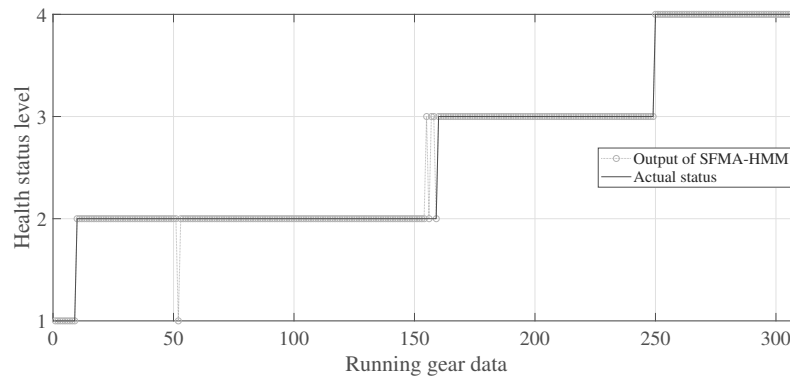
Fig. 11. SFMA simulation results.
