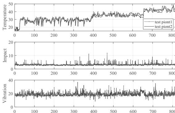
Fig. 7. Raw data.
