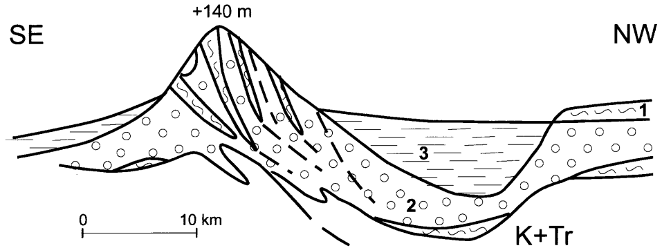
Rys.3. Przekrój depresji Quakenbrück i grzbietu Dammer w Dolnej Saksonii [Meyer, 1987]. Objaśnienia: K+Tr – kreda jeziorna i trzeciorzęd; 1 – gliny zwałowe; 2 – inne osady starszych zlodowaceń (głównie piaski); 3 – osady zbiornikowe (m.in. jeziorne) złożone w depresjach, głównie z interglacjalu eemskiego i zlodowacenia wistły.
