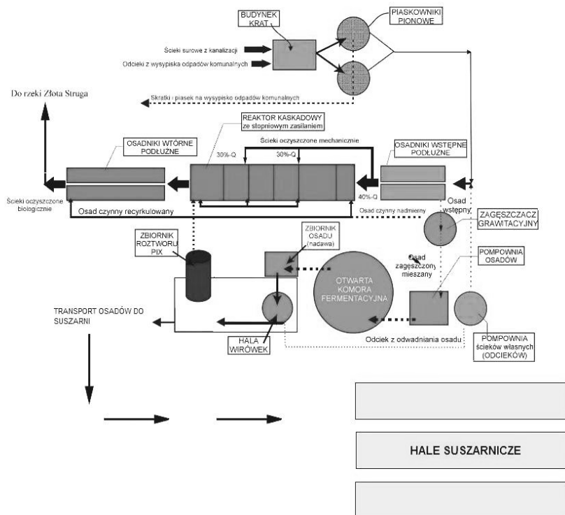
Rys. 1 Układ technologiczny oczyszczalni ścieków Złota Struga
