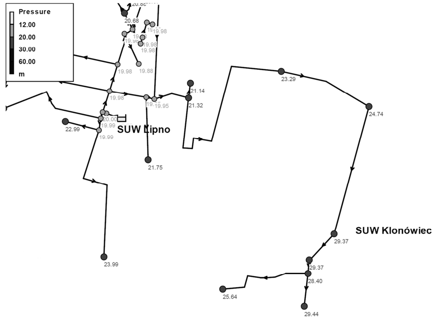
Rys. 14. Ciśnienie w sieci: połączenie Lipno-Klonowice - wersja 1 Fig. 14. Pressure in the network: connection Lipno-Klonowice - version 1
