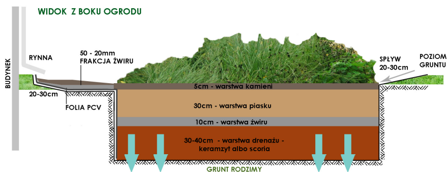
Rys. 2 Przekrój przez ogród deszczowy w gruncie, bez uszczelnienia dna – woda infiltruje do gruntu [Domanowska dla Fundacji Sendzimir]
