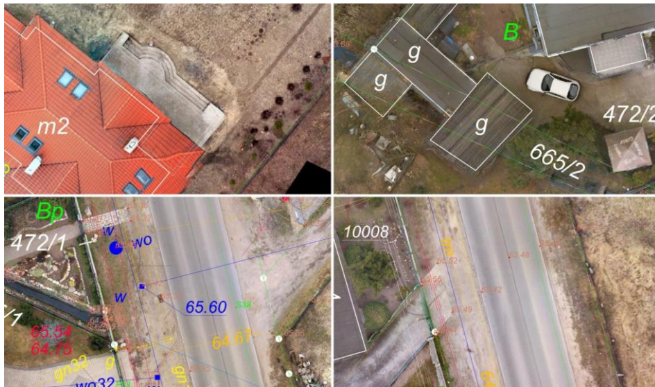
Rys. 4. Graficzne porównanie wyników opracowania fotogrametrycznego z UAV (pułap 60 m, kamera Sony a6000) z mapę wektorową uzupełnioną o bezpośredni pomiar punktów techniką GNSS/RTN nawiązanych do sieci ASG EUPOS. (źródło: opracowanie własne)
